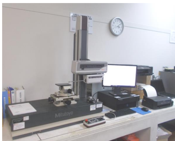
輪郭形状測定機
